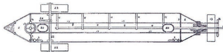
Tv. Snittegning af ubåden "Hunley", lavet på basis af konstruktionstegningerne. U.S. Naval Historical Center, foto NH 58769.
