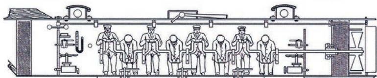
Top. Ubåden "Hunley". Tegning af R.G. Skerrett (1902) efter maleri C.W. Chapman fra 1863-64.
